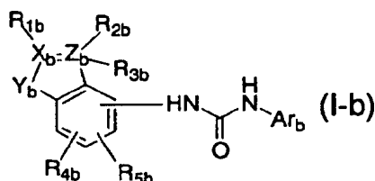
Formula (I-b)
